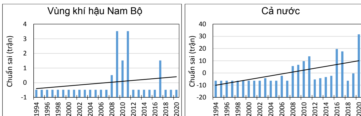
Hình 1.19. Diễn biến, xu thế số trận mưa đá xảy ra trên các vùng khí hậu giai đoạn 1994-2020
