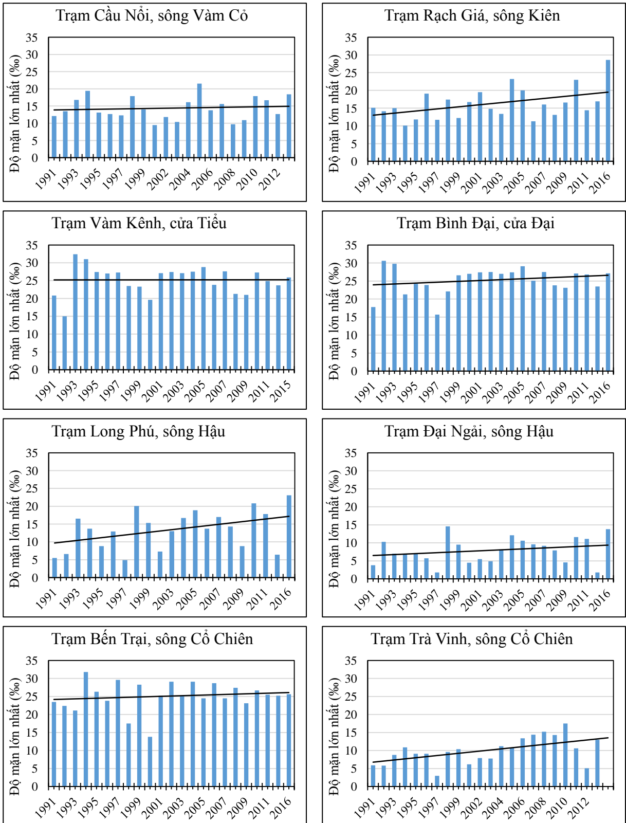
Hình 1.11. Diễn biến, xu thế độ mặn lớn nhất tại một số trạm thuộc vùng Nam Bộ
