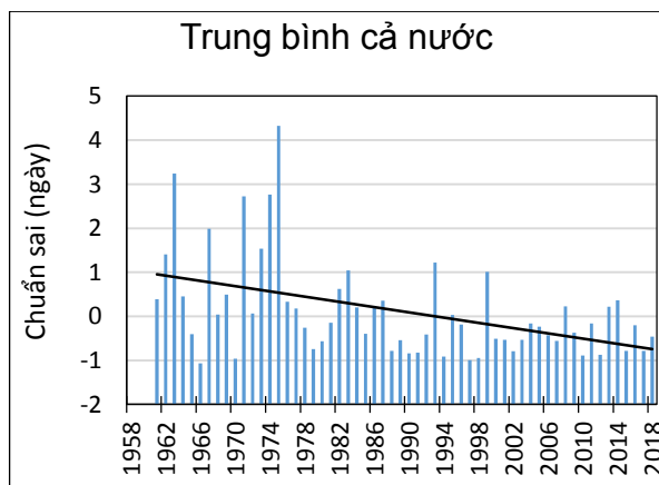
Hình 1.21. Diễn biến, xu thế số ngày sương muối tiềm năng xảy ra trên các vùng khí hậu giai đoạn 1961-2018
