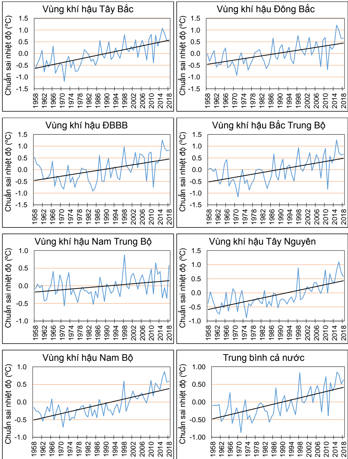
Hình 1.3. Diễn biến, xu thế nhiệt độ trung bình các vùng khí hậu
