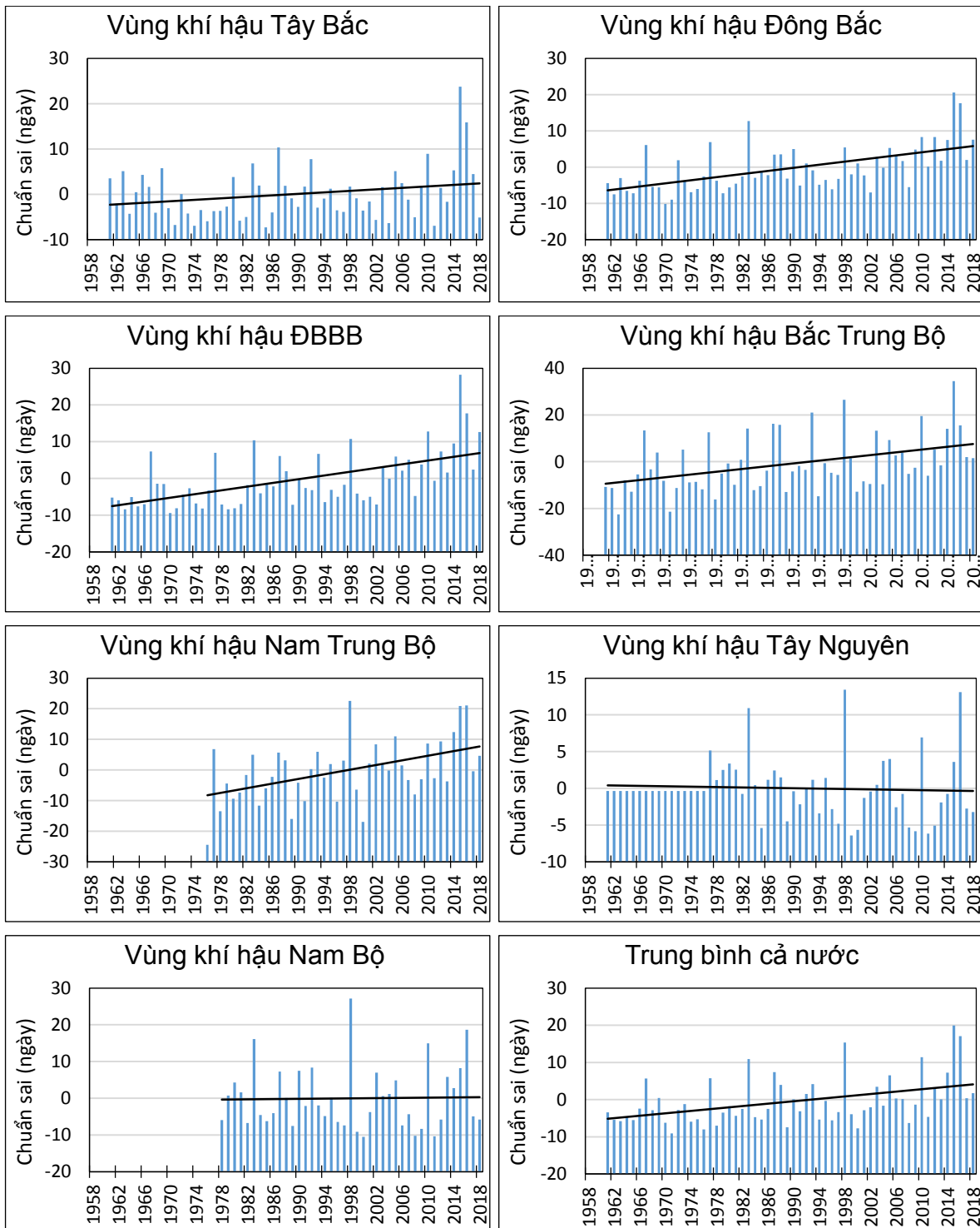
Hình 1.16. Diễn biến, xu thế số ngày nắng nóng xảy ra trên các vùng khí hậu giai đoạn 1961-2018
