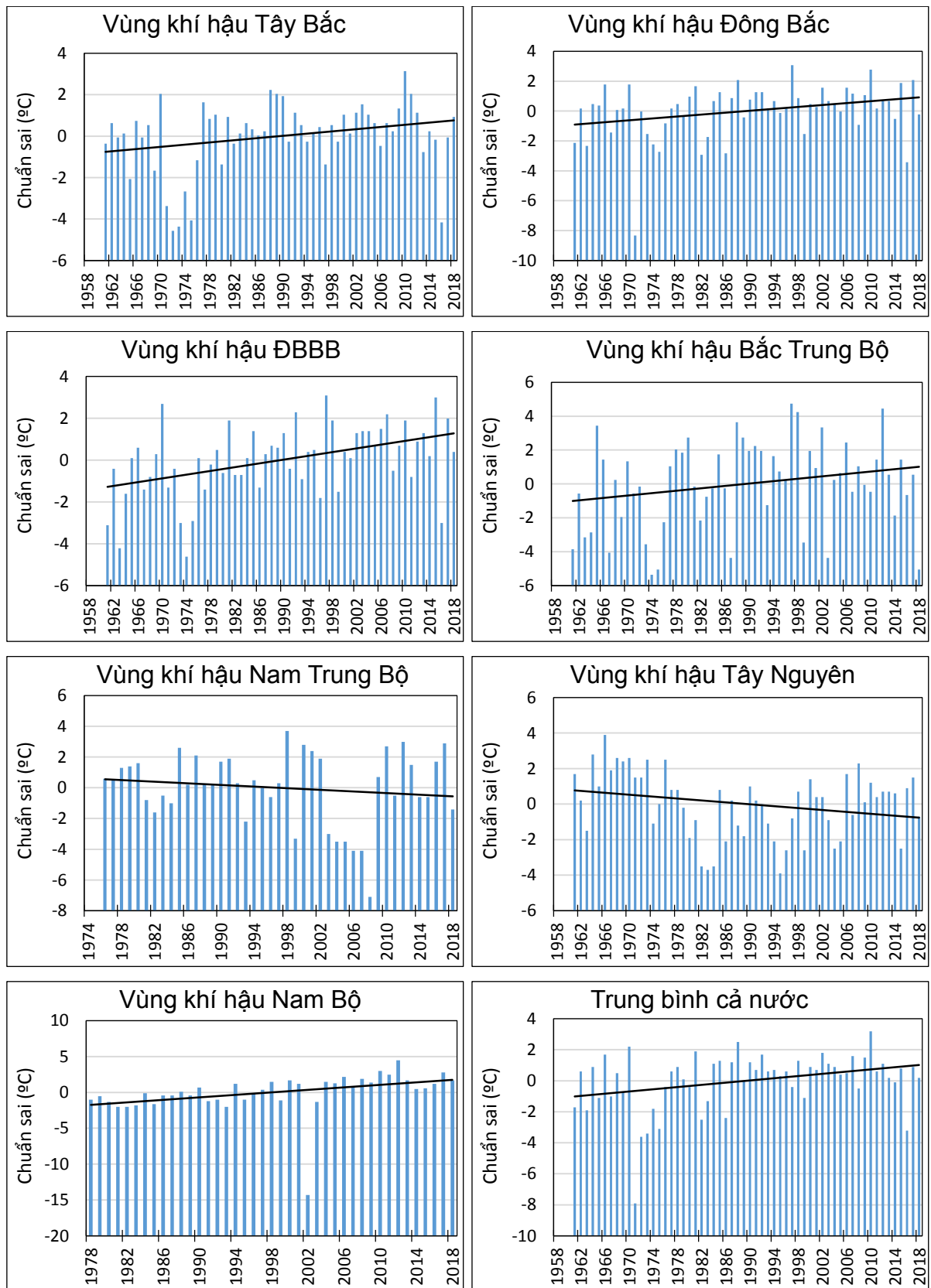
Hình 1.7. Diễn biến, xu thế nhiệt độ tối thấp tuyệt đối các vùng khí hậu Bảng 1.17. Kết quả kiểm nghiệm thống kê và đánh giá xu thế biến đổi nhiệt độ tối thấp tuyệt đối
